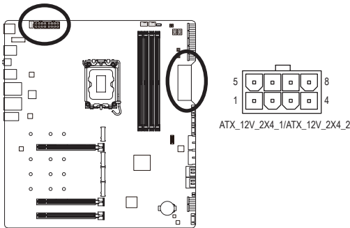
ATX_12V_2X4_1/ATX_12V_2X4_2:
